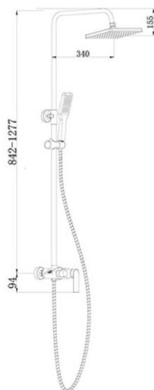
Стойка душевая
