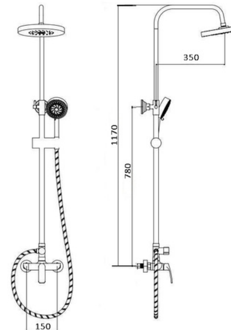
Стойки душевые
