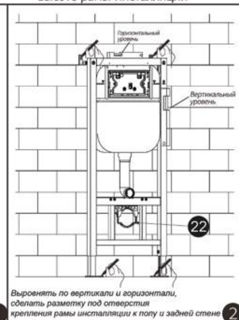
Монтаж в фальшстену по высоте рамы инсталляции
