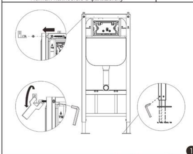
Монтаж полностью в фальшстену
